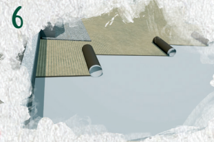
6 Colocar la malla SOLDRAIN (perpendicular a los rollos de césped) para el control de las malas hierbas y un drenaje óptimo
