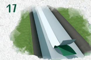
17 Opción 2: levantar los bordes (15-20 cm). Colocar cinta adhesiva TAPEFIX
